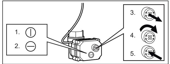
Kuva 18: 1. Pystyviiva osoittaa venttiilin olevan auki 2. Vaakasuora viiva osoittaa venttiilin olevan kiinni 3. Vedä nuppi suoraan ulos 4. Avaa/sulje venttiili kääntämällä nuppia 5. Palaa automaattiseen tilaan painamalla nuppia
