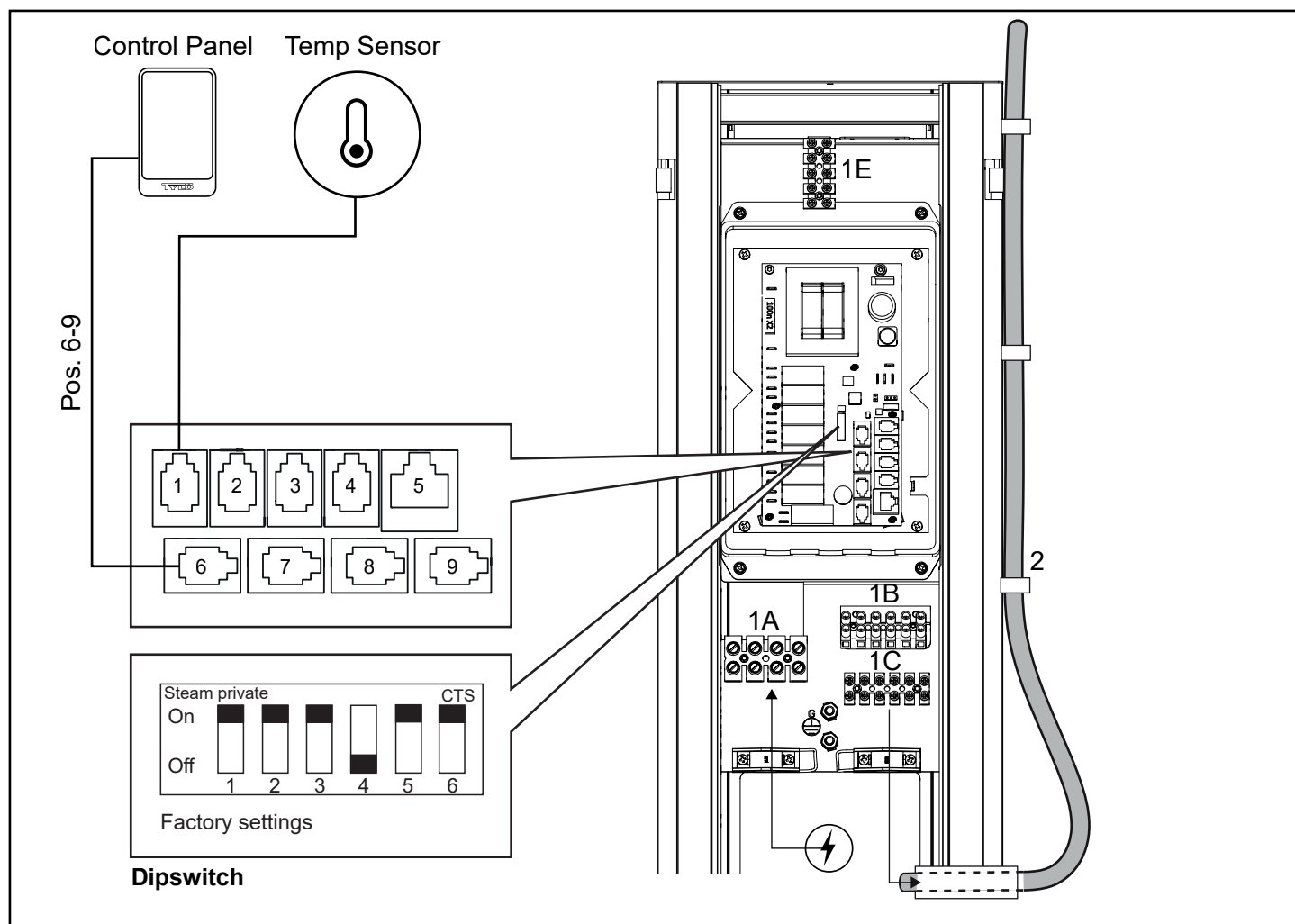
Рис. 5. Схема установки парогенератора Stella
