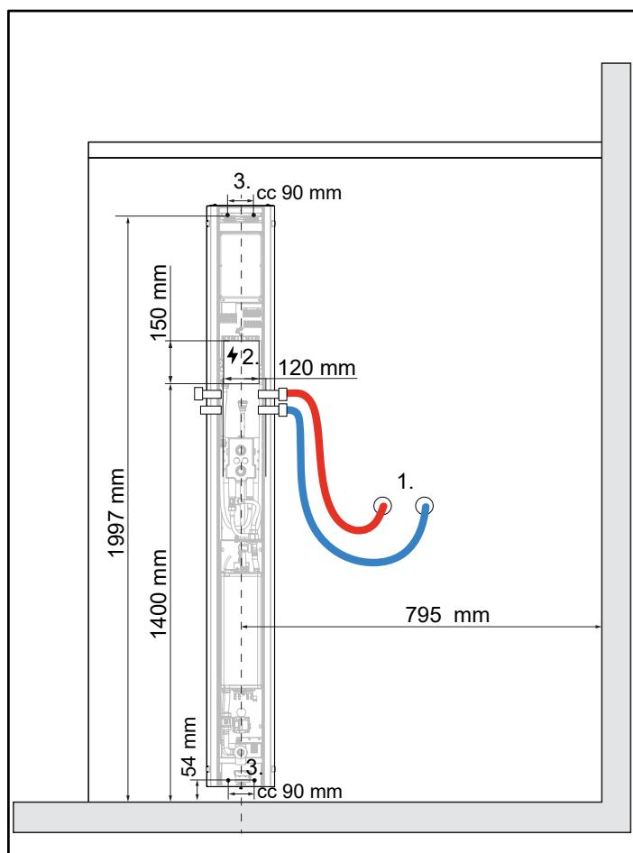
Kuva 4 Liittimet
