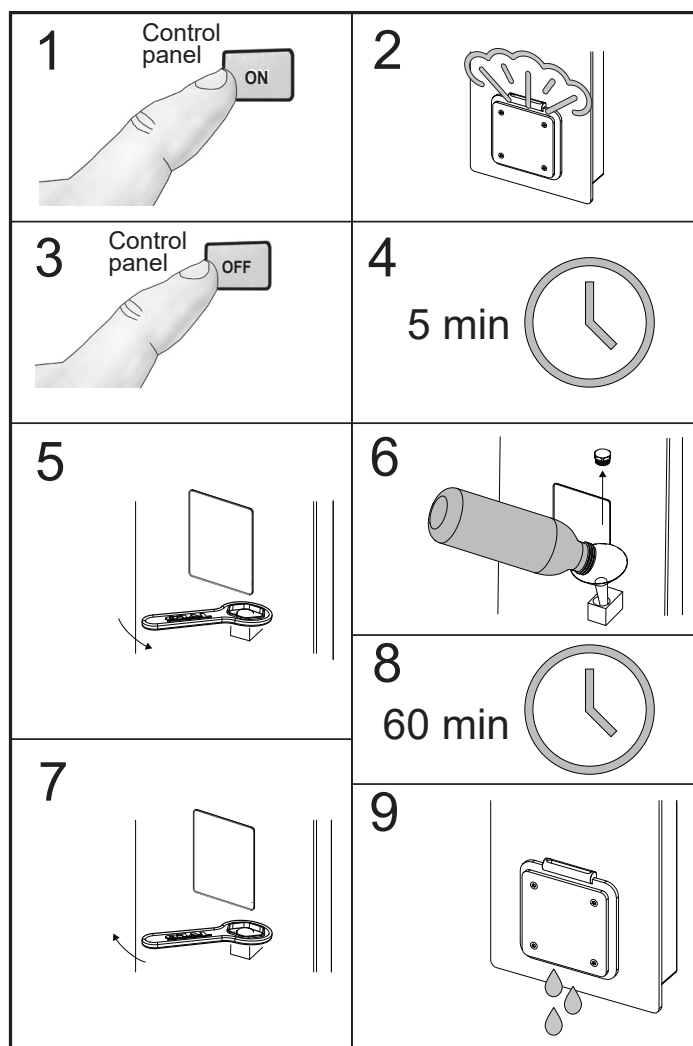
Fig. 12 Följ de olika stegen vid avkalkning av ånggeneratoren
