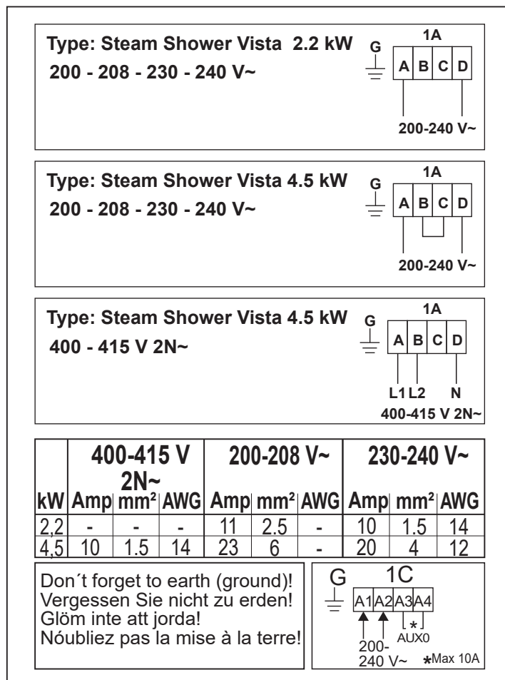
Abb 7. Anschlussplan
