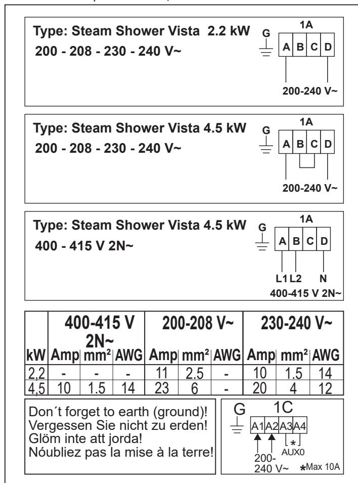
Рис. 7 Схема соединений
