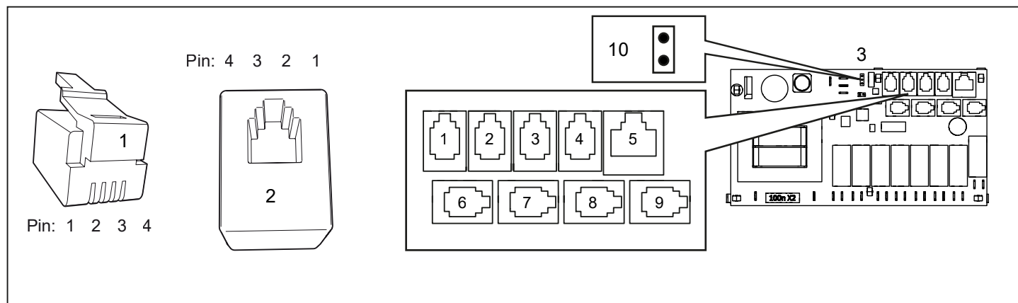
Рис. 10 Модульный штекер / модульный контактор и релейная плата
