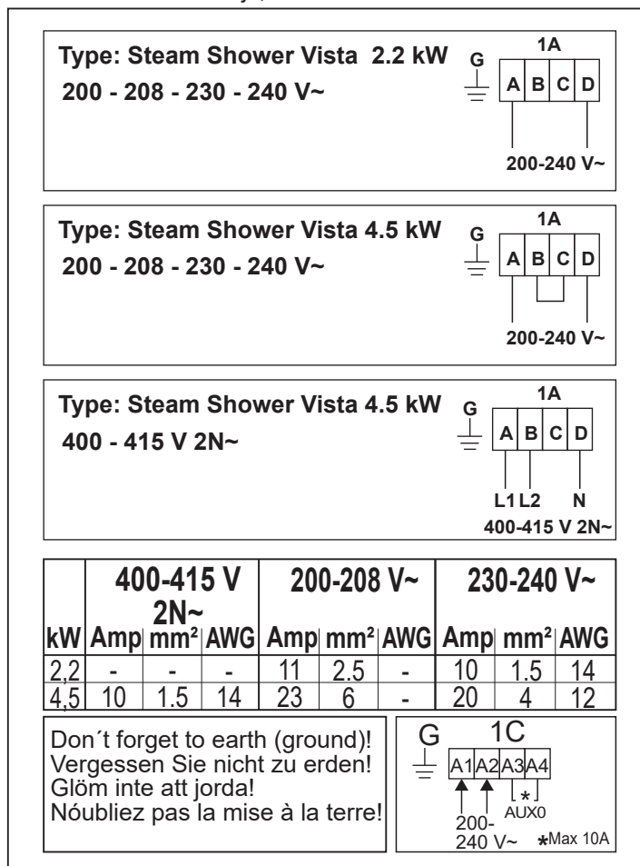
Kuva 7 Liitântäkaavio
