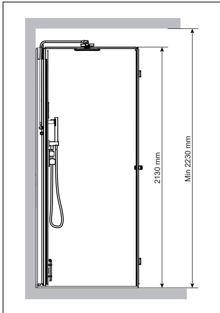
Figure 2 : Dimensions de la hauteur Vista
