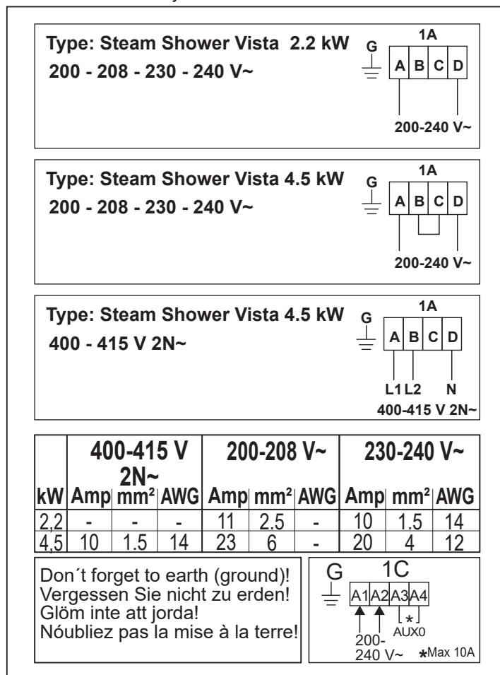
Fig. 7 Inkopplingsschema
