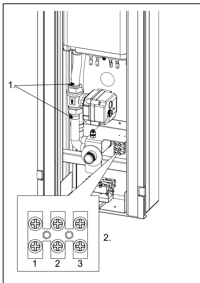
Abb. 19 Ersetzen eines defekten motorbetriebenen Kugelventils
